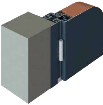
POSE EN BORDS TABLEAU Dormant étroit sans aile + plat de finition
