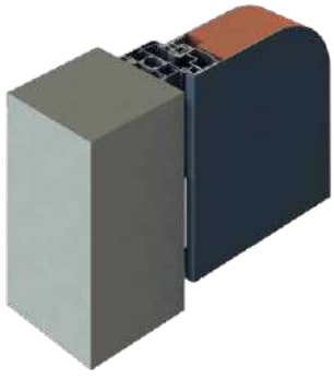
POSE EN TUNNEL Dormant intermédiaire sans aile
