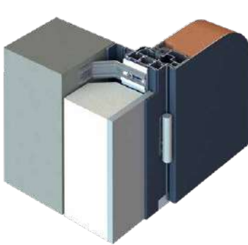
POSE EN APPLIQUE Dormant intermédiaire sans aile + tapée de doublage
