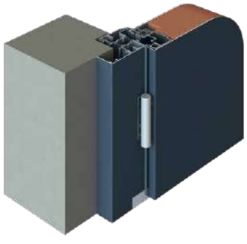
POSE EN FEUILLURE Dormant large sans aile + compensateur de feuillure
