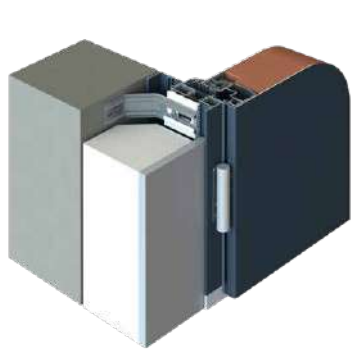
POSE EN APPLIQUE Dormant avec aile de 9 mm + tapée de doublage
