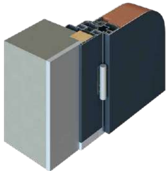
POSE EN RENOVATION SUR DORMANT EXISTANT Dormant avec aile de 60 mm + cornière de finition extérieure
